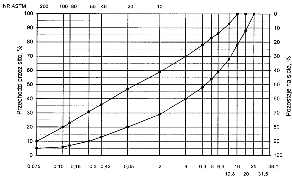
Rys. 1. Krzywe graniczne uziarnienia mieszanki mineralnej BA od 0 do 20 mm do warstwy ściaralnej nawierzchni drogi o obciążeniu ruchem dla KR2
