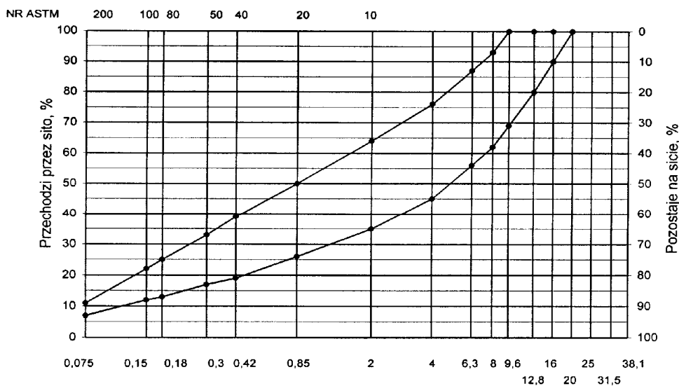
Rys. 2. Krzywe graniczne uziarnienia mieszanki mineralnej BA od 0 do 16mm, od 0 do 12,8 mm do warstwy ściaralnej nawierzchni drogi o obciążeniu ruchem KR2
