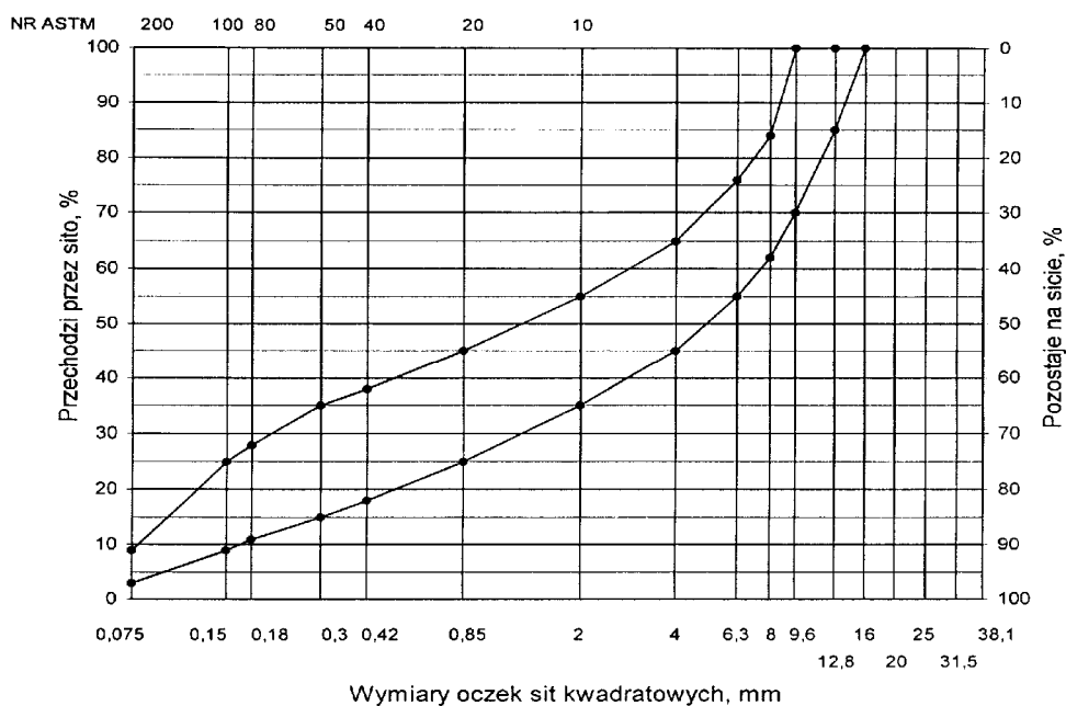
Rys. Krzywe graniczne uziarnienia mieszanki mineralnej BA od 0 do 12,8 mm do warstwy wiążącej, wyrównawczej i wzmacniającej nawierzchni drogi o obciążeniu ruchem KR2
