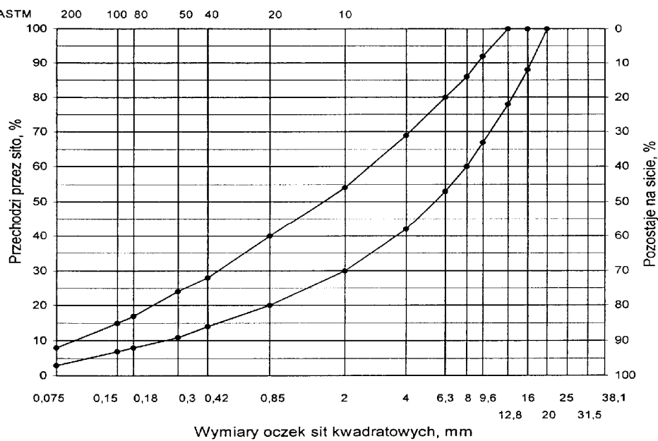
Rys. Krzywe graniczne uziarnienia mieszanki mineralnej BA od 0 do 16 mm do warstwy wiążącej, wyrównawczej i wzmacniającej nawierzchni drogi o obciążeniu ruchem KR2
