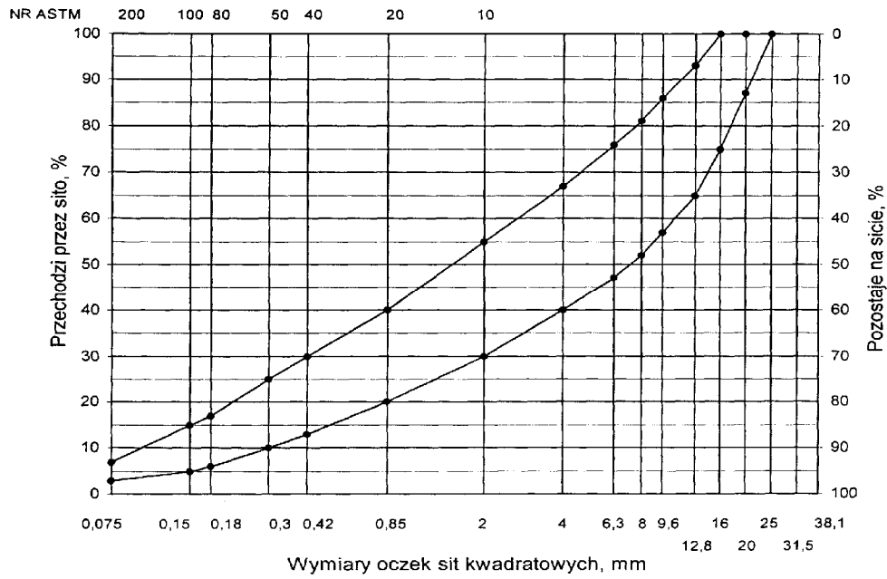
Rys. Krzywe graniczne uziarnienia mieszanki mineralnej BA od 0 do 20 mm do warstwy wiążącej, wyrównawczej i wzmacniającej nawierzchni drogi o obciążeniu ruchem KR2
