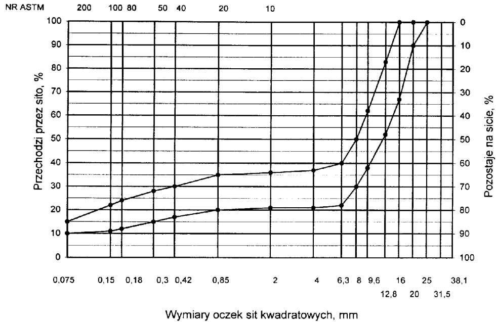
Wymiary oczek sit kwadratowych, mm Rys. 5. Krzywe graniczne uziarnienia mieszanki mineralnej BA od 0 do 20 mm (mieszanka o nieciągłym uziarnieniu) do warstwy ścieralnej nawierzchni drogi o obciążeniu ruchem od KR3 do KR6
